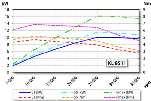
Güç diyagramı
